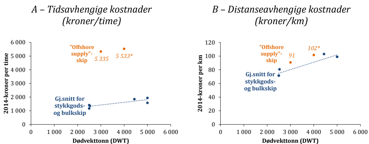
Figur 5.4 Predikerte tids- og distanseavhengige kostnader for et «offshore supply»-skip på 4000 DWT, 2016-kroner
