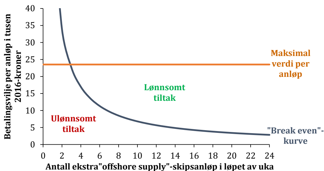
Figur 6.2 «Break even»-kurve med maksimal verdi per anløp
