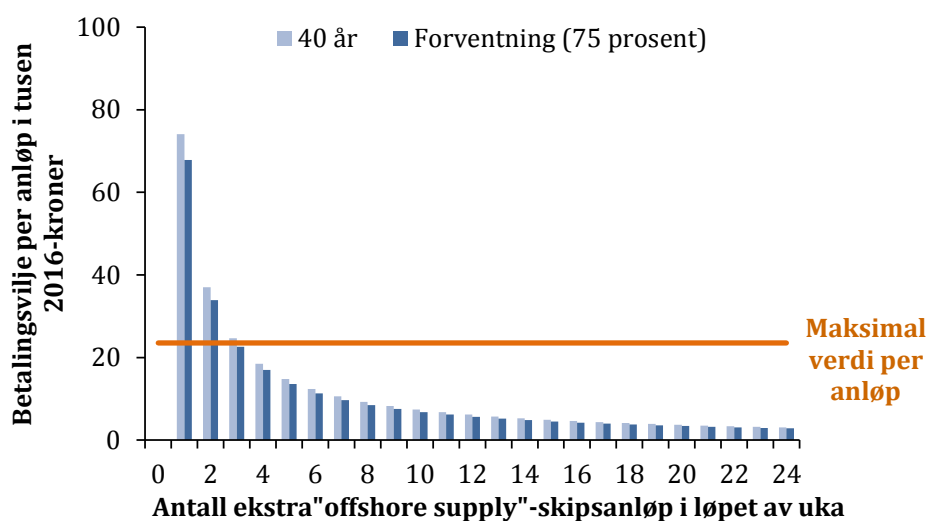
Figur 6.5 Nødvendig betalingsvilje per anløp for ulike omfang av ekstra «offshore supply»-skipsanløp, med ulik levetid
